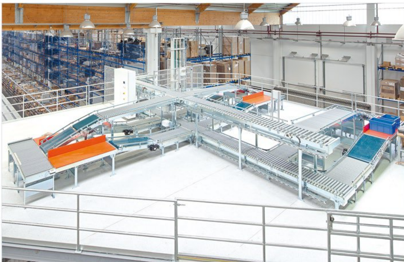
4-Packplatz-Anlage mit Kontrolltischen bei einem Online-Händler.
