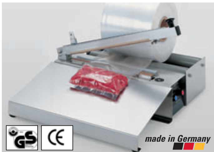
HPL 300 mit Anbautisch und Folienabrollgerät
